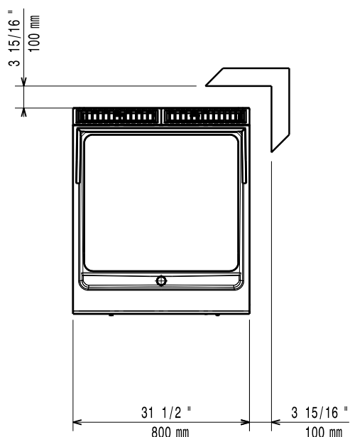
Felülnézet
