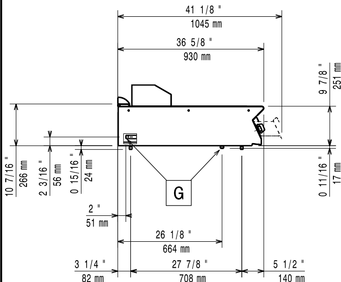
Oldalnézet
